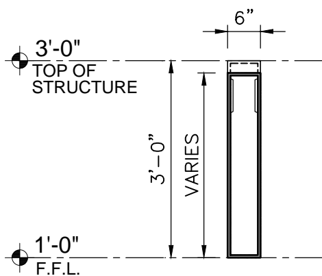
SECTION A SCALE: 1/2" = 1'
