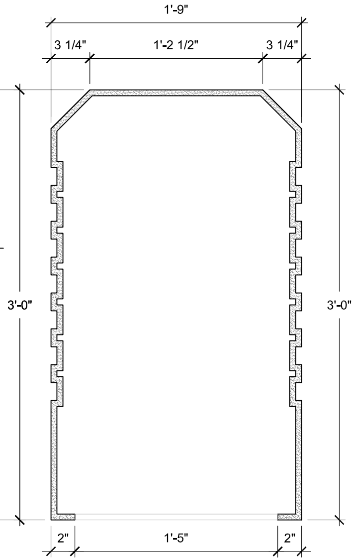
SECTION B SCALE: 1 1/2" = 1'-0"
