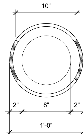
SECTION B SCALE: 1 1/2" = 1'-0"
