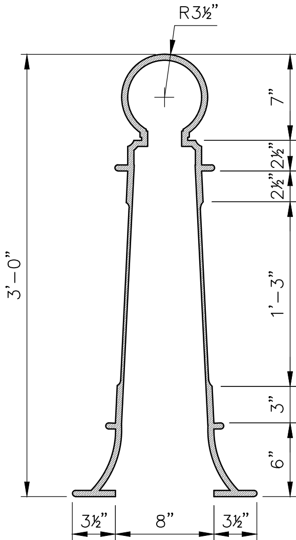
SECTION A SCALE: 1-1/2" = 1'
