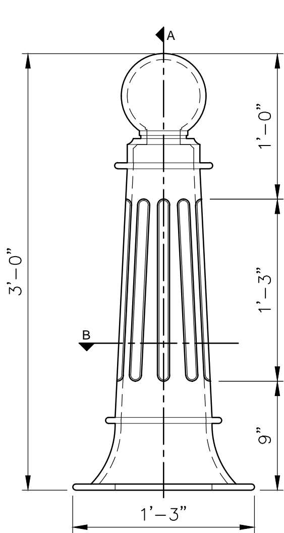
FRONT ELEVATION SCALE: 1-1/2" = 1'
