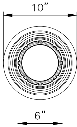
SECTION B SCALE: 1-1/2" = 1'
