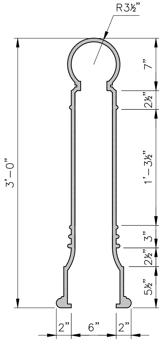
SECTION A SCALE: 1-1/2" = 1'
