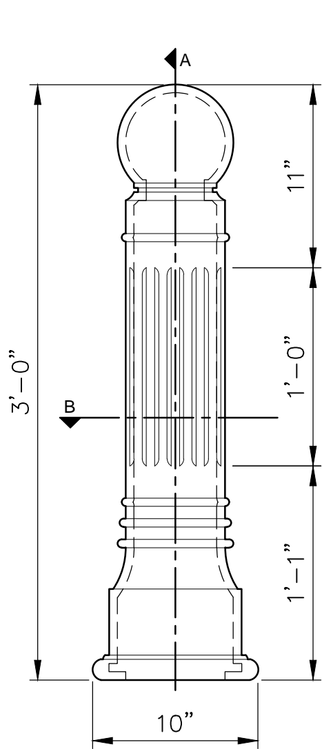
FRONT ELEVATION SCALE: 1-1/2" = 1'
