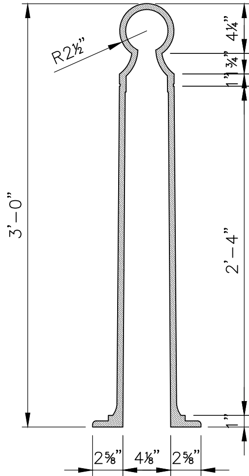
SECTION A SCALE: 1-1/2" = 1'
