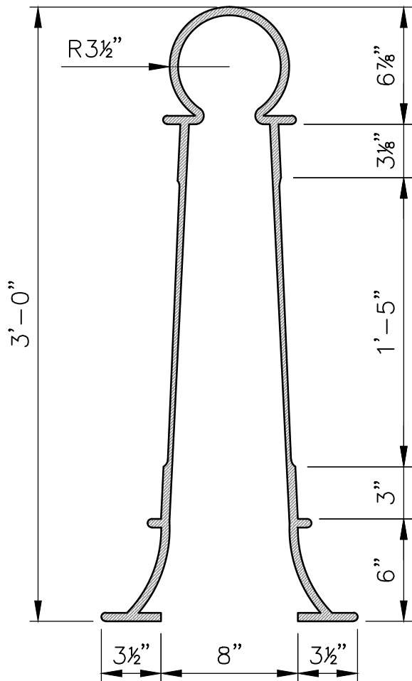
SECTION A SCALE: 1-1/2" = 1'
