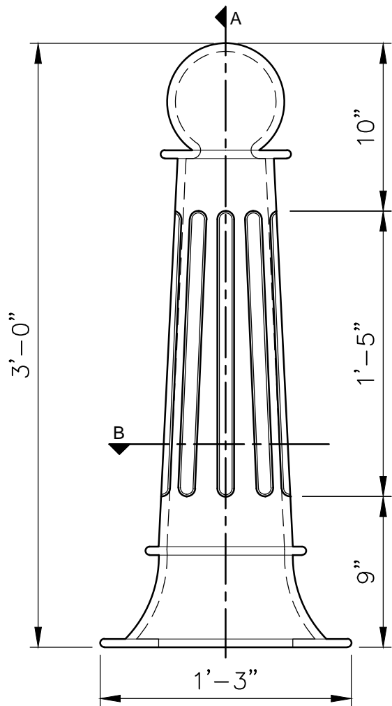
FRONT ELEVATION SCALE: 1-1/2" = 1'
