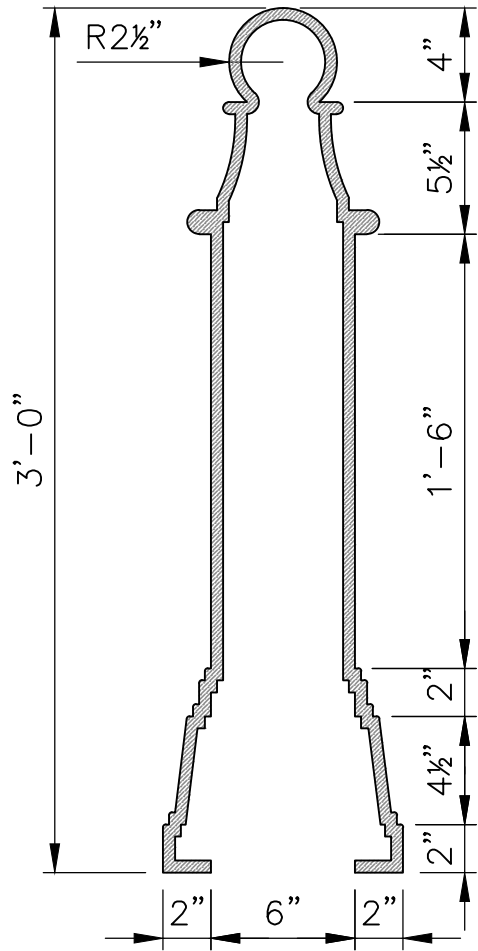
SECTION A SCALE: 1-1/2" = 1'
