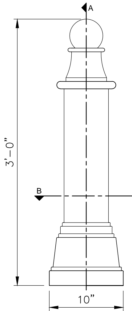
FRONT ELEVATION SCALE: 1-1/2" = 1'
