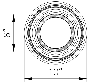
SECTION B SCALE: 1-1/2" = 1'
