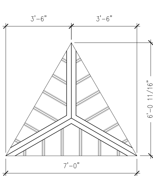
TOP VIEW SCALE: \frac{3}{8}" = 1'-0"
