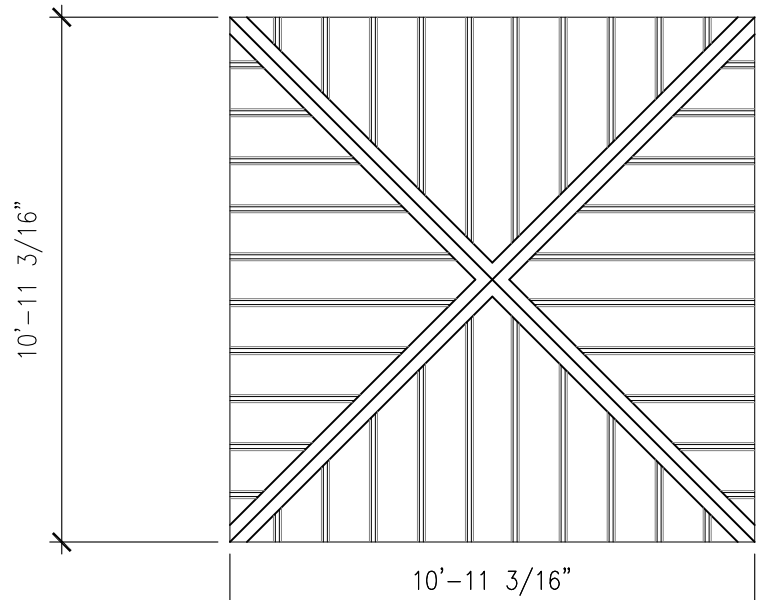
TOP VIEW SCALE: 1/4" = 1'-0"
