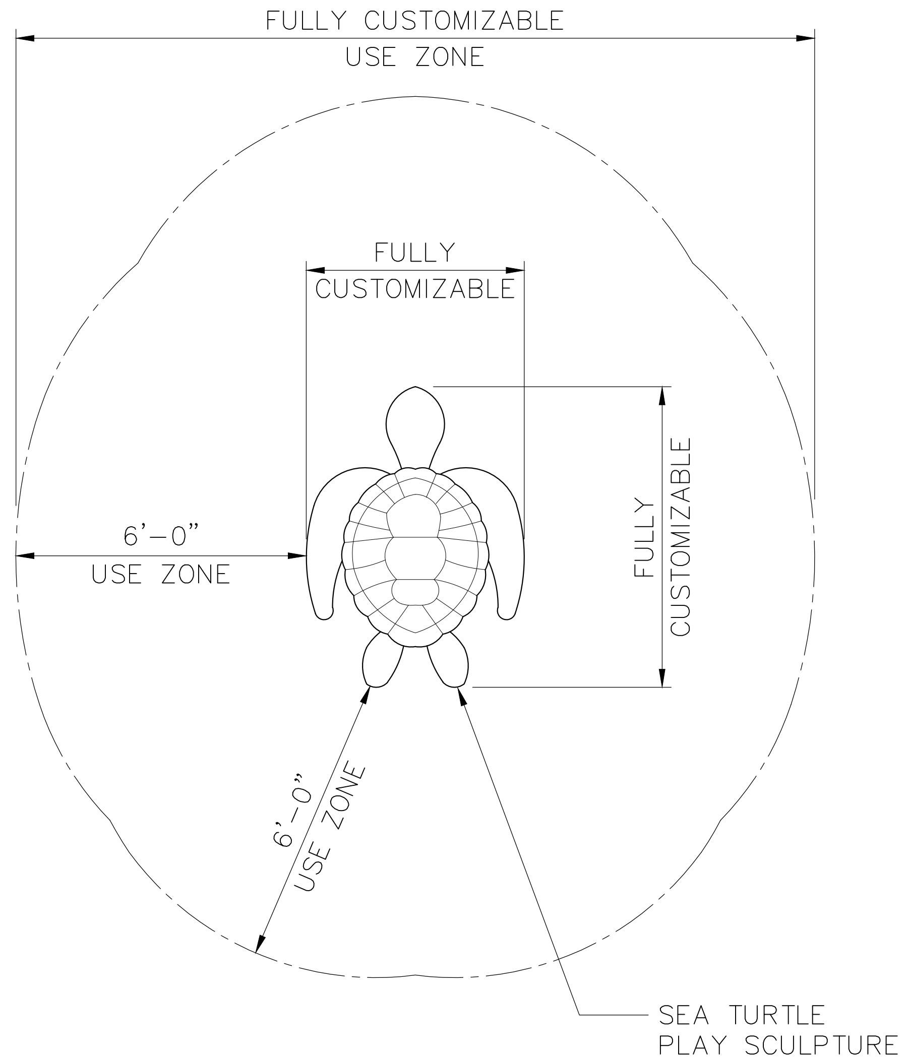
TOP VIEW SCALE: 1/2" = 1'-0"
