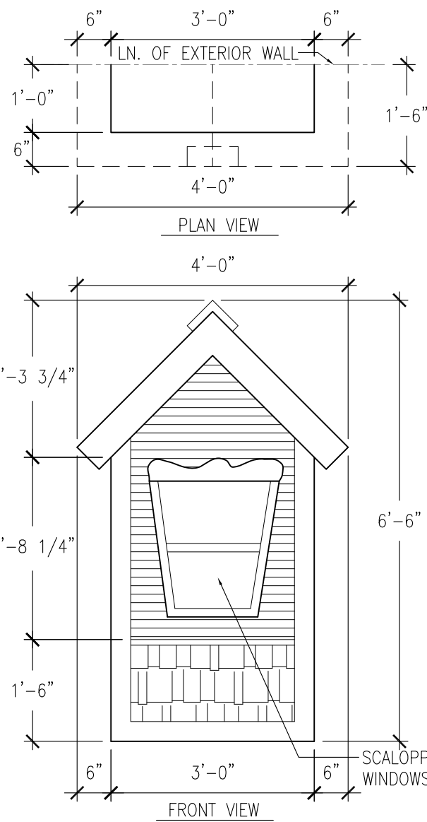
DORMER 02
