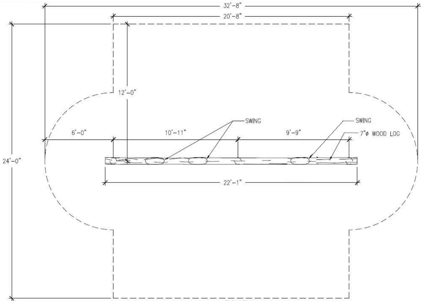
TOP VIEW SCALE: 1/4" = 1'-0"
