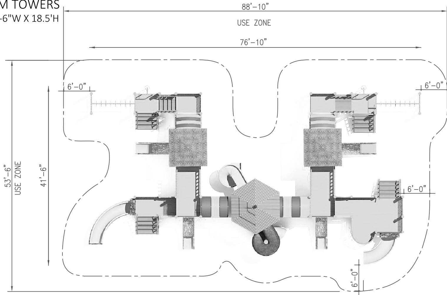
TOP VIEW SCALE: 1/2" = 1'-0"
